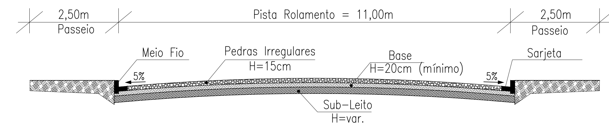
Perfil Topográfico Esquemático da Avenida Esc: s/esc.
